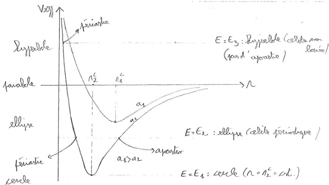
FIGURE 7.1 – Représentation du potentiels pour de différentes valeurs d'énergie.
